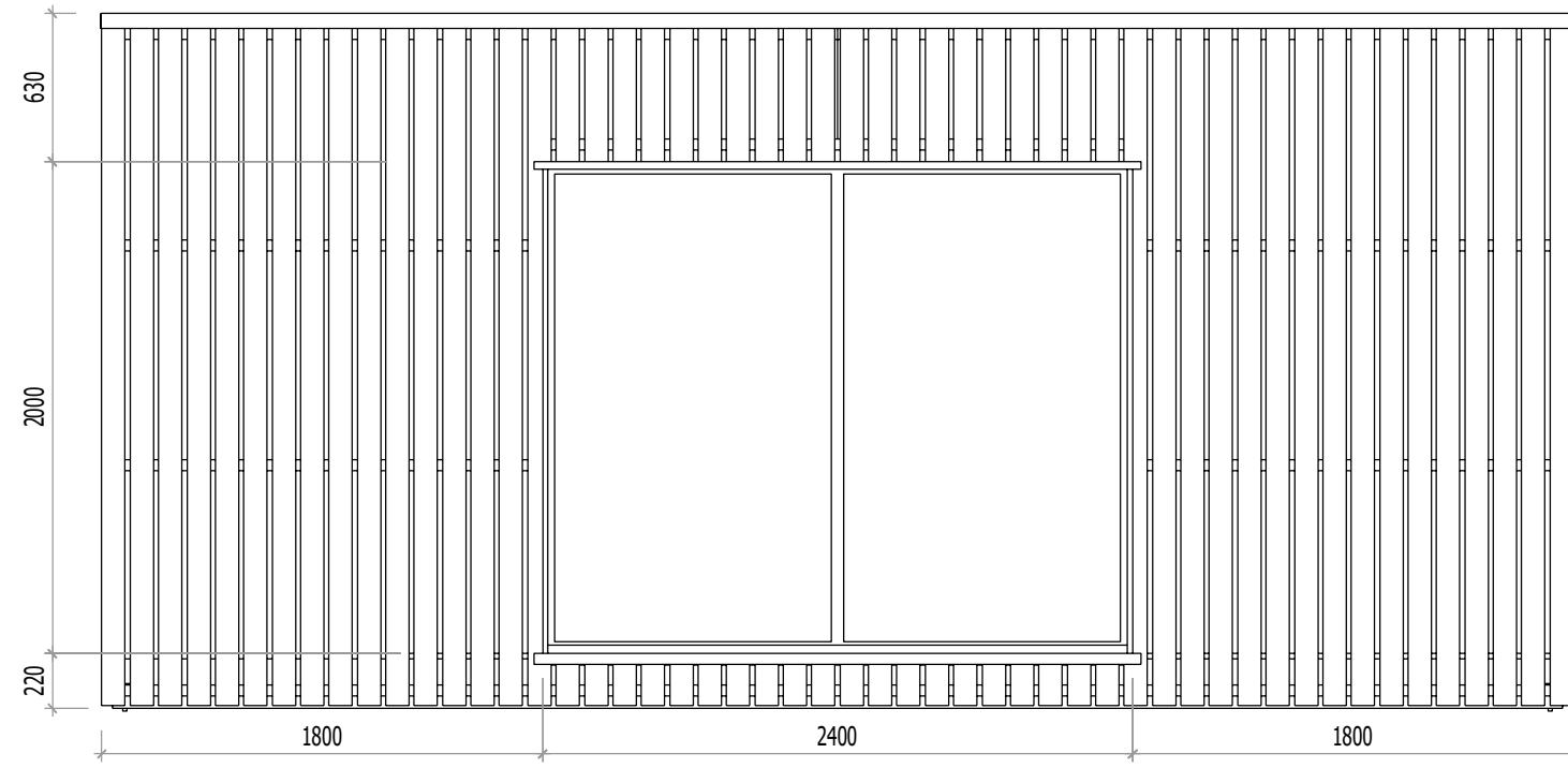
VUE FACE AVANT
